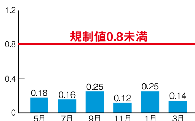
フッ素及びその化合物 2024 (mg/L)
